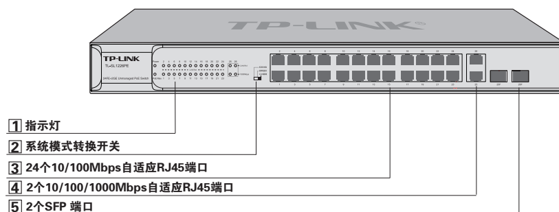
图1-4 TL-SL1226PE前面板示意图
