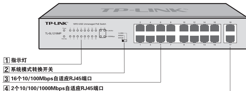
图1-2 TL-SL1218MP前面板示意图
