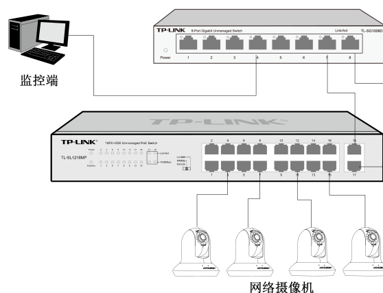
图1-5 视频监控模式连接拓扑图
