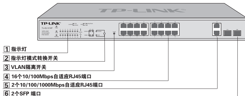
图1-1 TL-SL1218P前面板示意图
