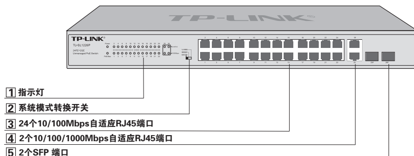
图1-3 TL-SL1226P前面板示意图
